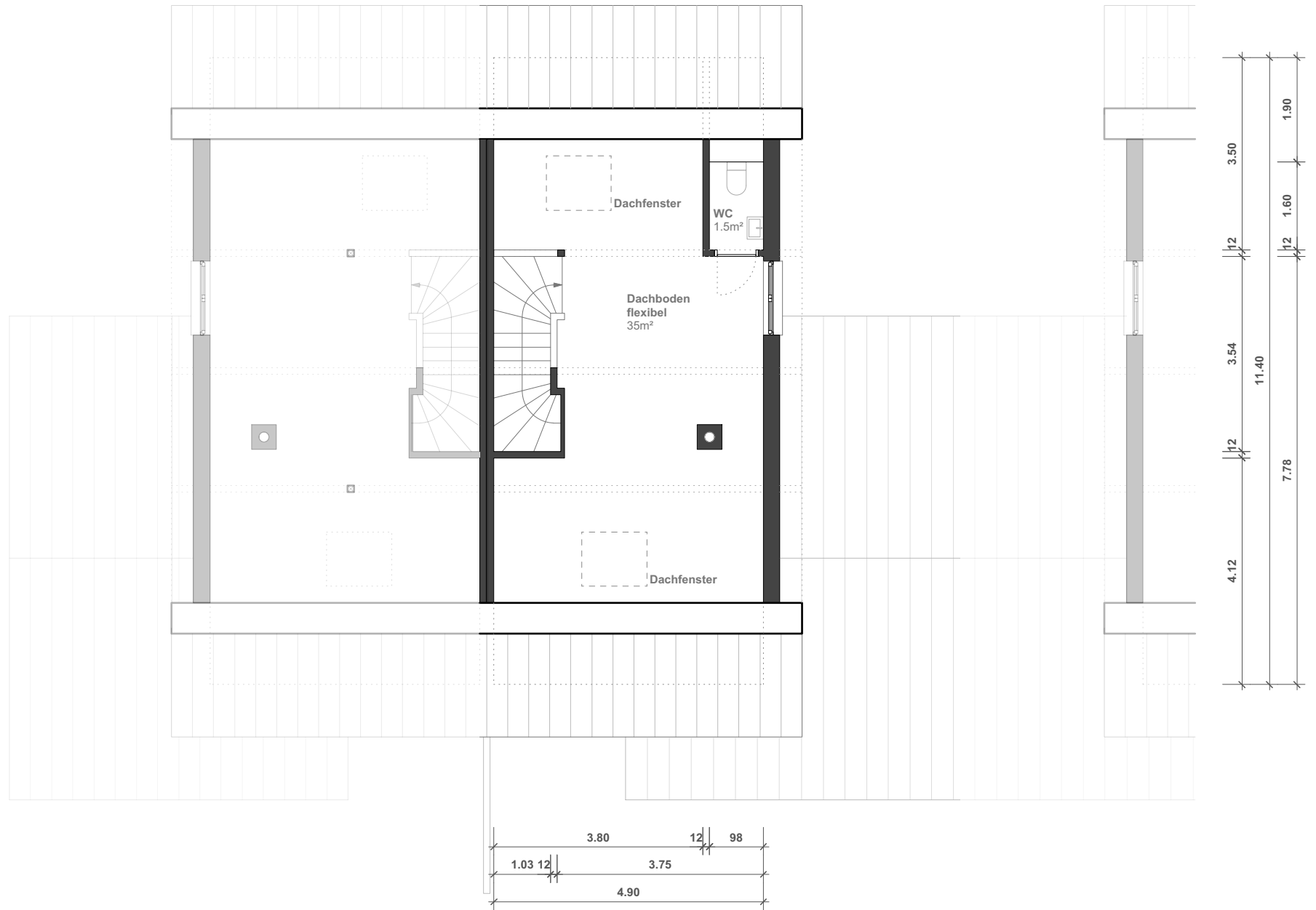
Grundriss DG M 1:100
